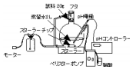
図 4 還流溶出試験装置
