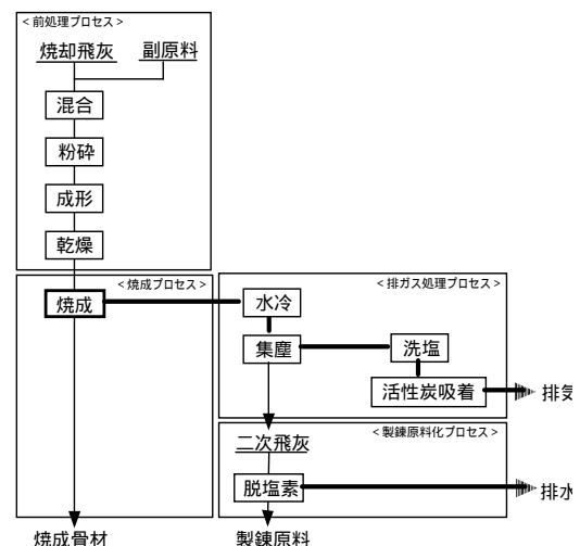
図1 焼成プロセス
