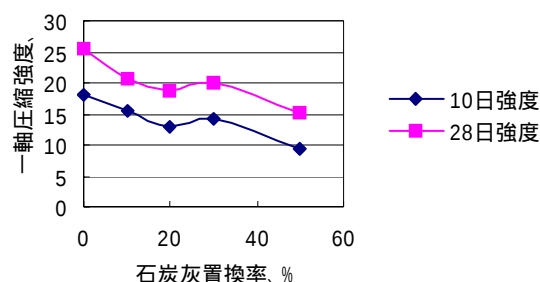
図 1 石炭灰置換率と強度の関係
