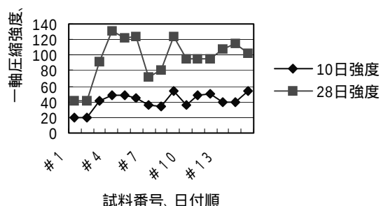
図 3 実機灰による強度の変化
