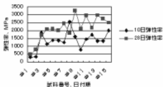
図 4 実機灰による弾性率の変化
